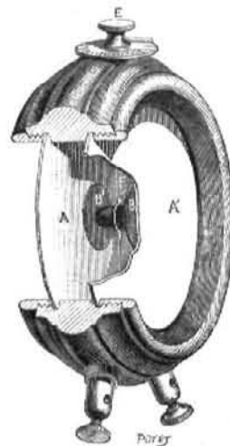
Fig. 2.—Micrófono de torsión
