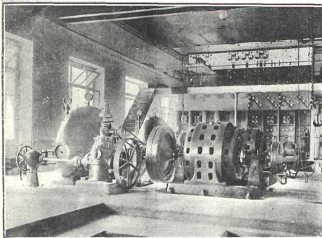
SALA DE MÁQUINAS DEL FERROCARRIL ELÉCTRICO.—CONDUCTORES AÉREOS DE LA ESTACIÓN DE PONTEBROLLA
