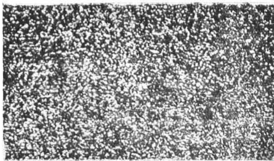
Estructura de la fotosfera: "Los granos de arroz".
