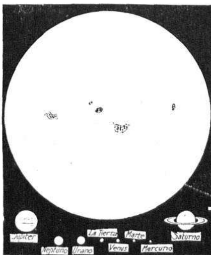
Dimensiones comparadas del Sol y de los principales planetas.
