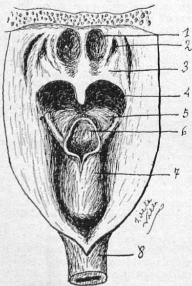
FARINGE ABIERTA POR SU CARA POSTERIOR. 1. Choanas.—2. Orificio de la trompa.—3. Velo del paladar.—4. Isthmo de las fauces.—5. Lengua.—6. Epiglotis.—7. Laringe.—8. Esófago
