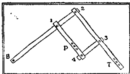
Vista detallada del pantógrafo
