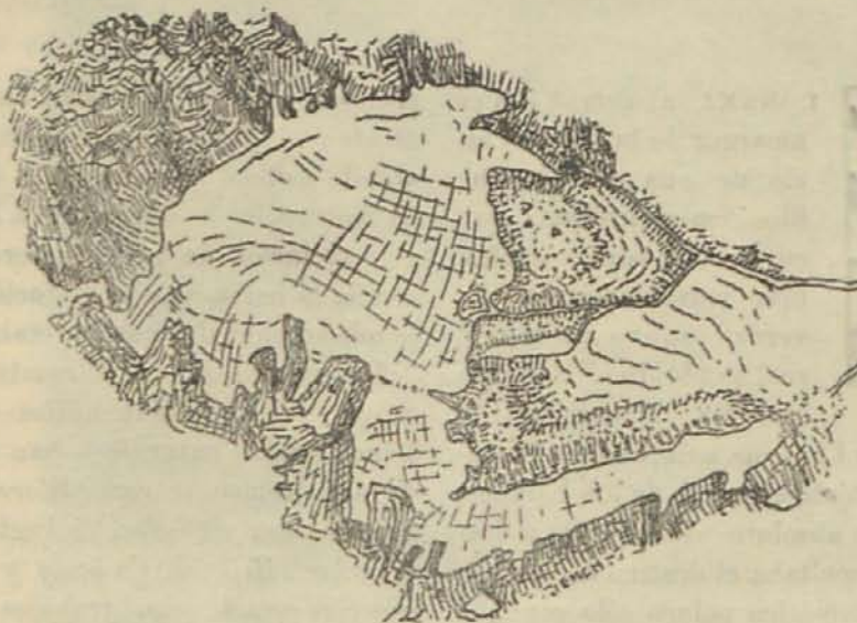
Grietas glaciares.
