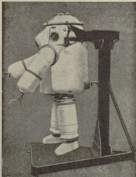
Fig. 4.—Aspecto exterior del equipo representado esquemáticamente en la figura 1.
