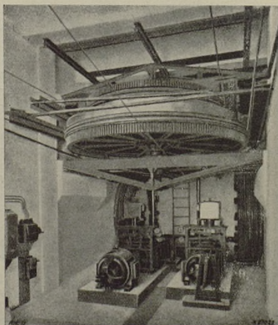
Fig. 4.—Sala de máquinas, accionamientos y tambores principal y auxiliar.
