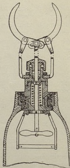
Fig. 3.—Indicación del accionamiento o de las manostenazas del equipo para grandes profundidades.
