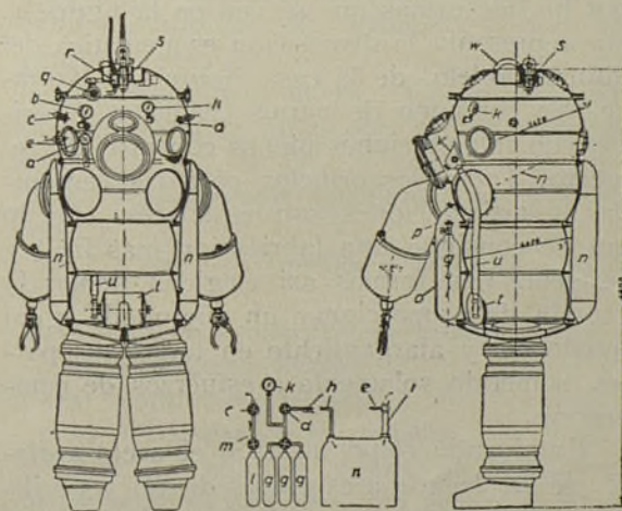
Fig. 1.—Disposición esquemática de un modelo de equipo blindado para buzos, que permite alcanzar profundidades de 150 metros.
