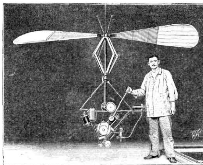
Fig. 2. - Un ensayo de aleo con un motor de petróleo
