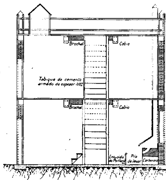
Corte vista. (Escala de 1 : 50.)
