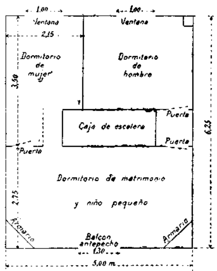
Distribución de habitaciones. Planta principal.
