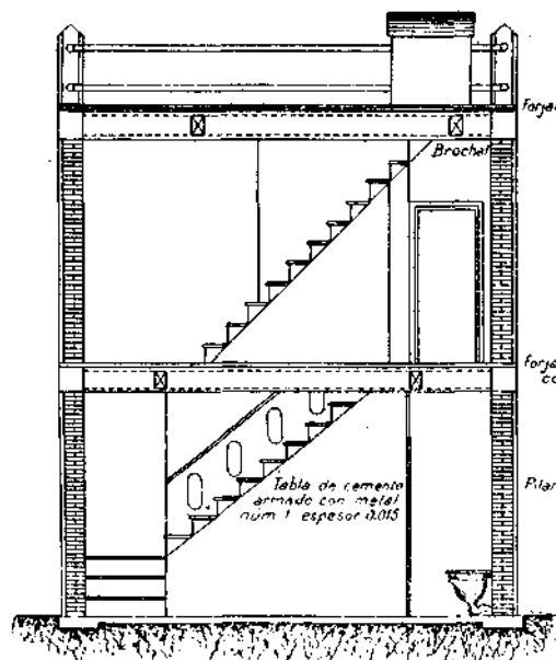
Corte vista. (Escala de 1 : 100.)
