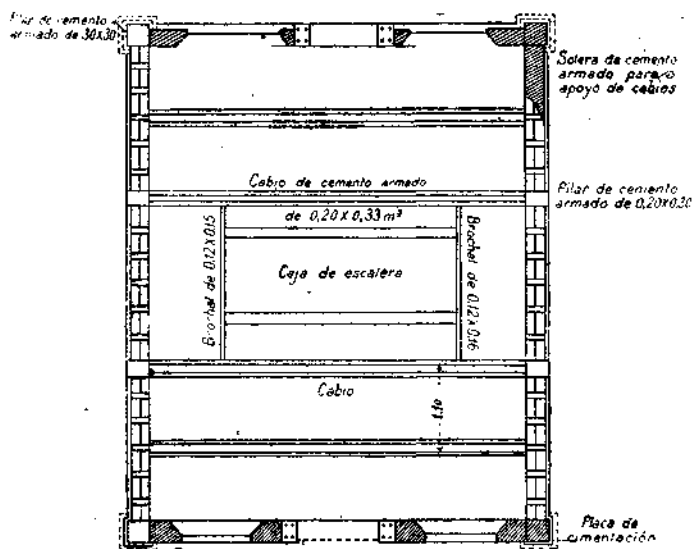
Planta cimientos. (Escala de 1 : 100).
