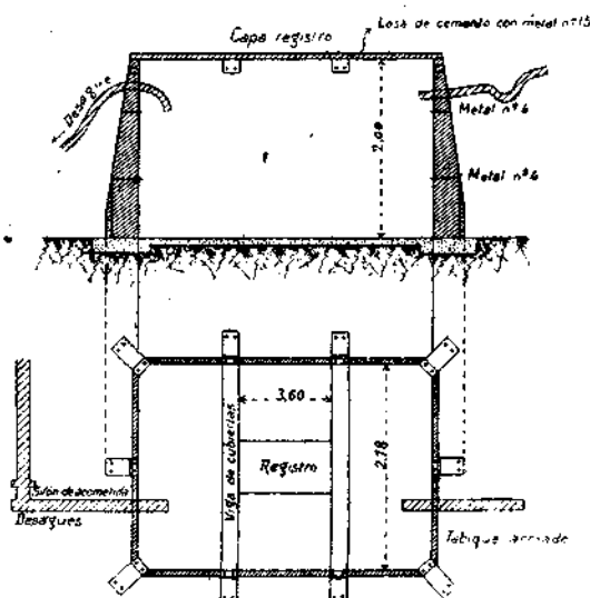
Pozo Mourás para 100 personas. Escala de 1 : 100.)
