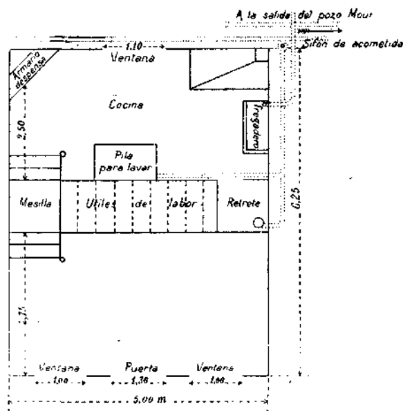
Distribución de habitaciones. Planta baja. (Escala de 1 : 50.)
