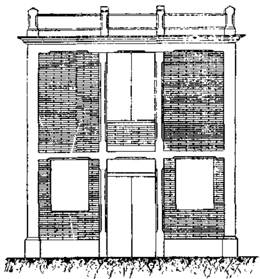
Vista de frente. Fachada principal. (Escala de 1 : 100.)
