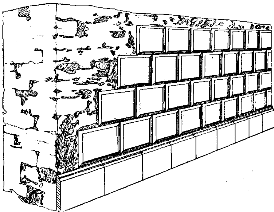
Revestimiento de un muro con piedra-vidrio.
