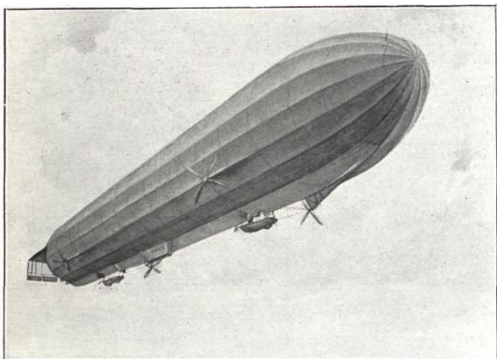
Dirigible alemán Z-VI , rígido, de 19,500 m. 3 ; longitud, 141 m.; diámetro, 14'8 m.; motores, 540 H. P.; velocidad, 77 kilóm. Construido en 1913
