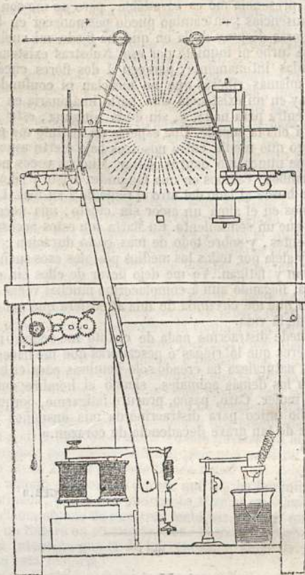
Luz eléctrica.—Aparato de M. Foulcaut. (V. la pág. 49.)
