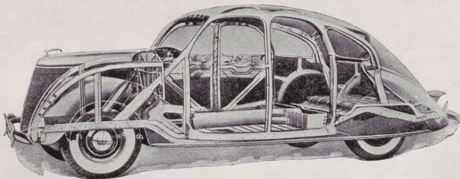
Diagrama de la construcción, enteramente de acero, del armazón de la carrocería del Zephyr de Lincoln. El esqueleto completo de la carrocería ocupa el lugar del bastidor corriente. Todas las piezas están unidas por soldadura, incluyendo las del piso. El techo de acero, los paneles laterales y los paneles traseros, lo mismo que el cubretablero, están unidos también por soldadura al armazón de la carrocería. Este tipo de esqueleto o bastidor ha despertado mucha atención entre los fabricantes de carrocerías, y se anticipa que similares construcciones se ofrecerán el próximo año por otros fabricantes.
