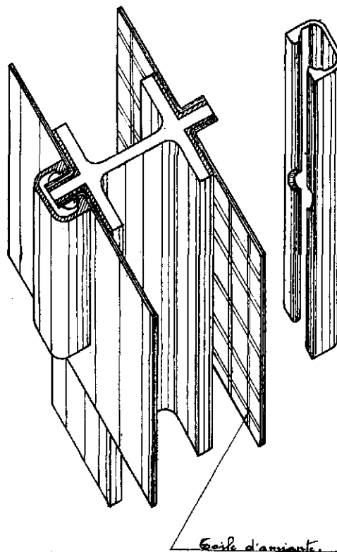
Detalle del montaje del tabique en el camarote "Stodal"
