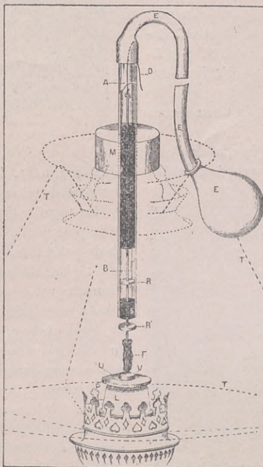
LÁMPARA DE MAGNESIO PARA OBTENER EFECTOS DE LUZ LOCALIZADA
