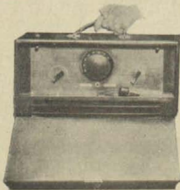
Aparato manual de dos lámparas
