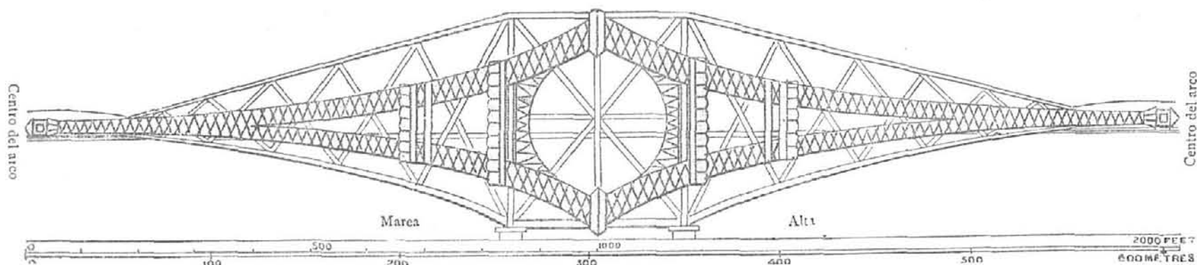
Figura 1. - Tamaño comparativo de dos torres Eiffel, puestas horizontalmente, con la viga equilibrada (cantilever) de Inchgarvie
